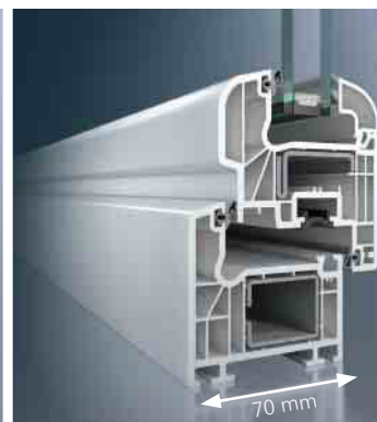
Hohe Basissicherheit: Die erhöhte Bautiefe und weit innen liegende Beschläge entziehen die Verschlusselemente dem Angriff der Einbrecher.
